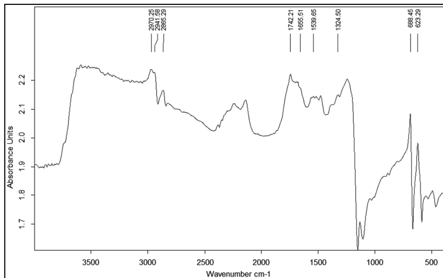
Fig. 13. Spectru FTIR
